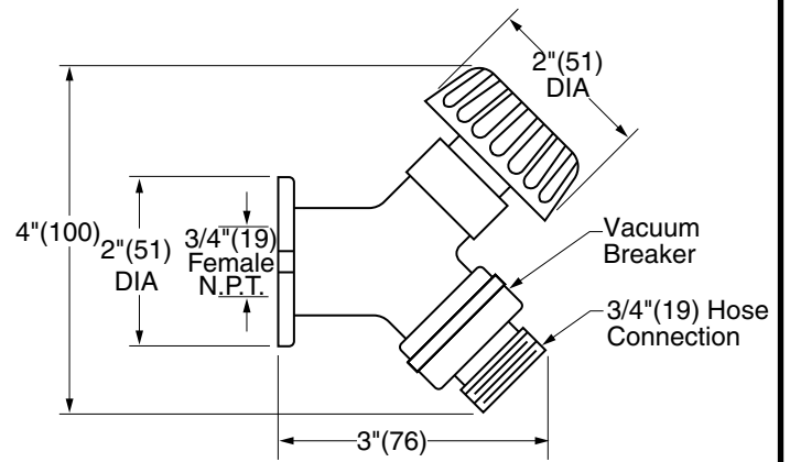
Fig. 5673.....3/4"(19) Inlet
